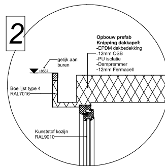
GEW. VOORGEVEL
