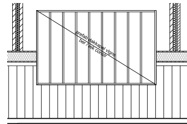
2e VERDIEPING PATDAKCONSTRUCTIE
