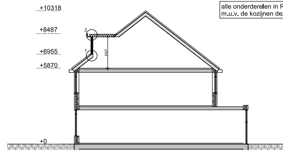
DWARSDOORSNEDE
