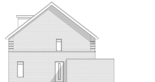
RECHTER ZIJGEVEL
